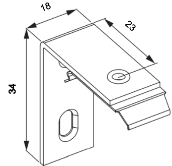
FACE FIX (Wall fix)
